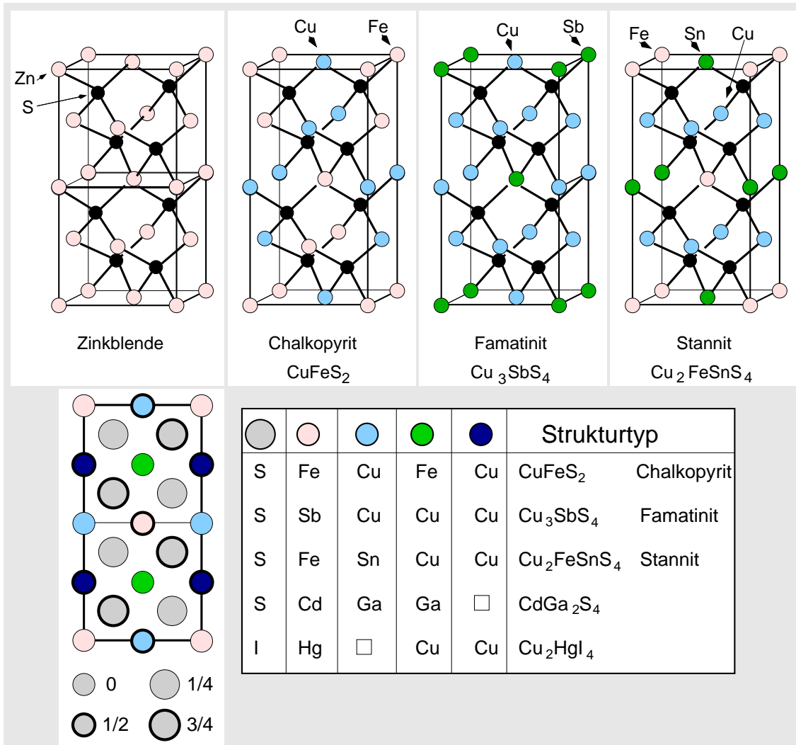
Überstrukturen der Zinkblende
