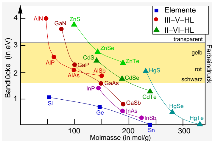
Bandlücken binärer Grimm-Sommerfeld-Verbindungen
