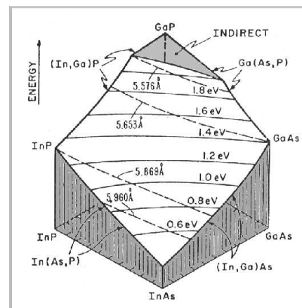
Verlauf der Bandlücke im quaternären System (In,Ga)(As,P)
