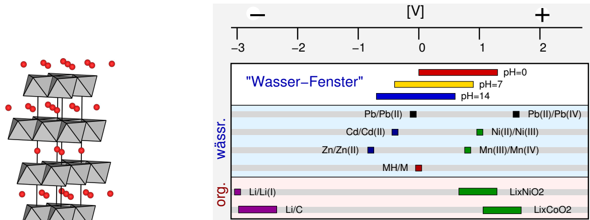
Potentiale von Elektrodenreaktionen in versch. Battersystemen
