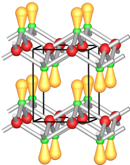
Struktur von PbO
