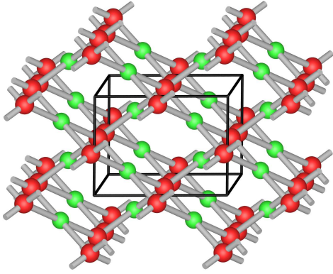
Struktur von CuO (Tenorit)
