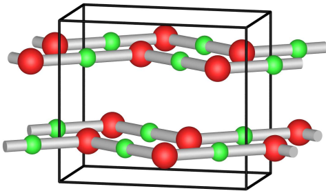
Struktur von HgO (rot)
