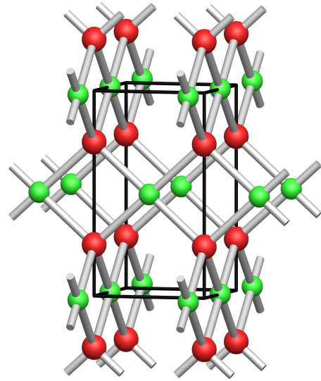
Struktur von PdO und PtS (PtS-Typ)
