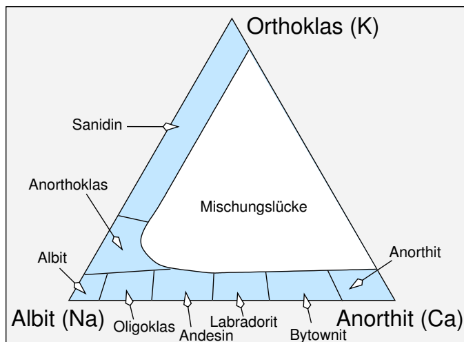
Mineralogische Namen und Phasenbreiten bei Feldspäten
