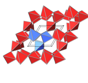
8.6. Feldspäte M I [AlSi 3 O 8 ] und M II [Al 2 Si 2 O 8 ]
