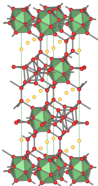
\text{RbGa}_7
