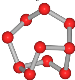
\text{Se}_{10}^{2+}
