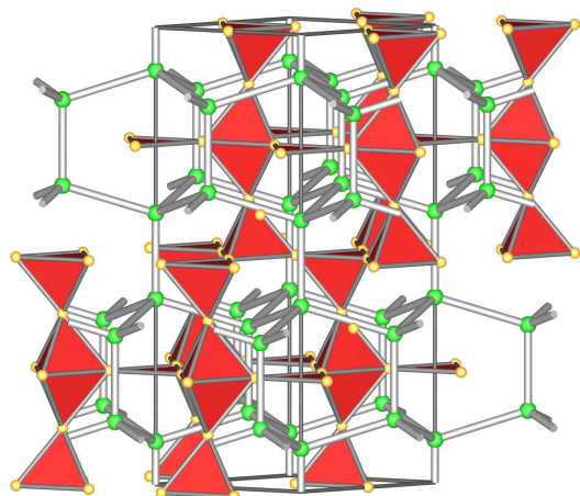
MgNi 2
