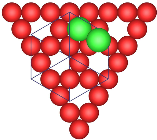
Cu-Kagomé-Netz
