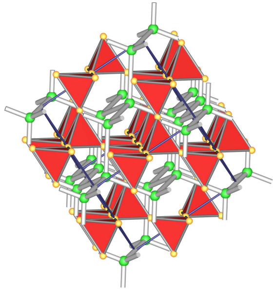
MgCu 2 : Gesamtstruktur
